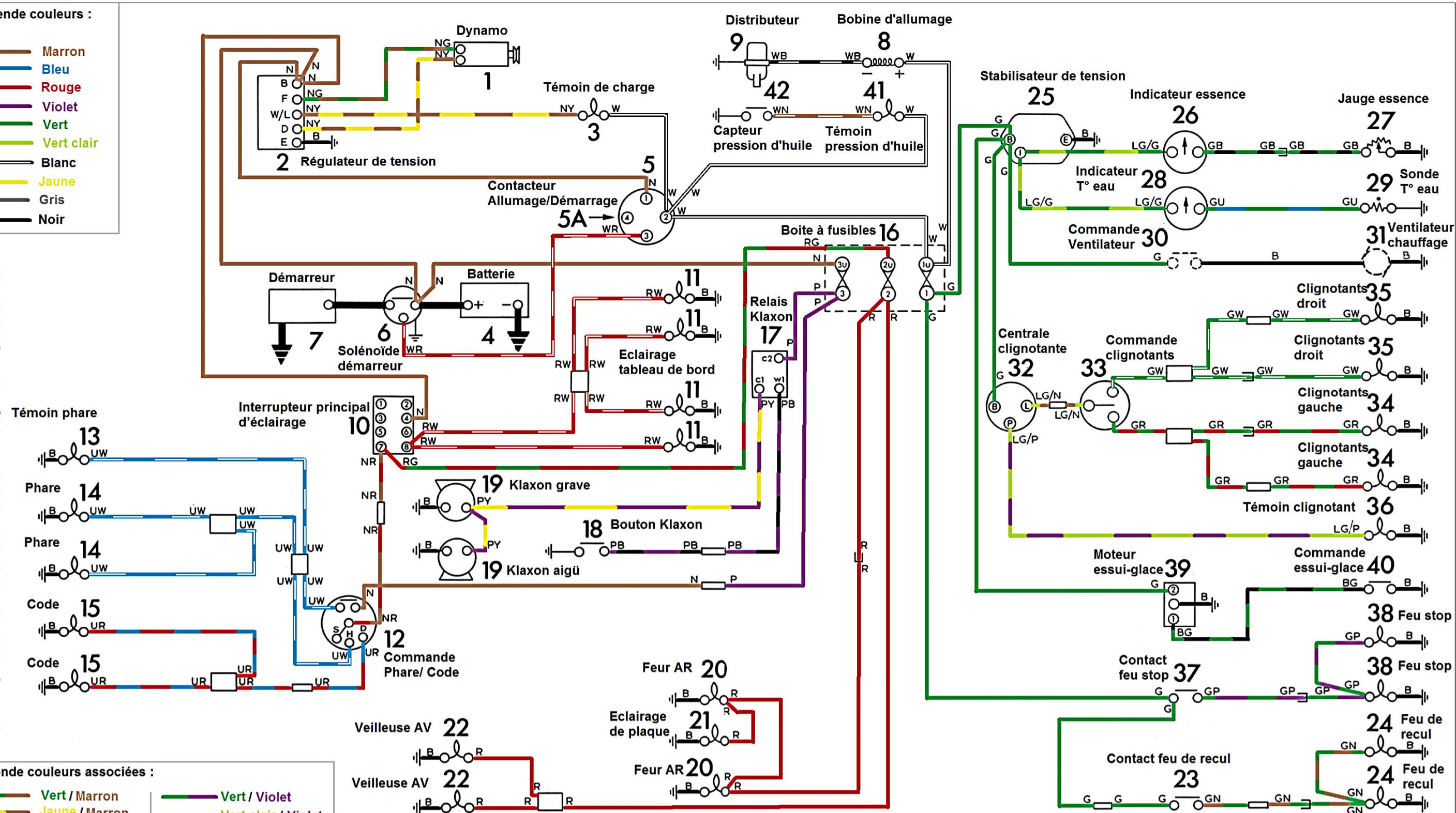
Fig. 4. Schéma de câblage - Spitfire Mark 3 - Conduite à gauche
