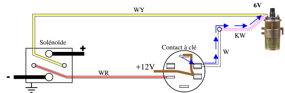
Schéma B position marche (Ignition)
