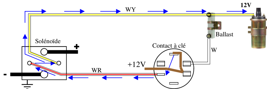
Schéma avec résistance ballast position démarrage (Start)
