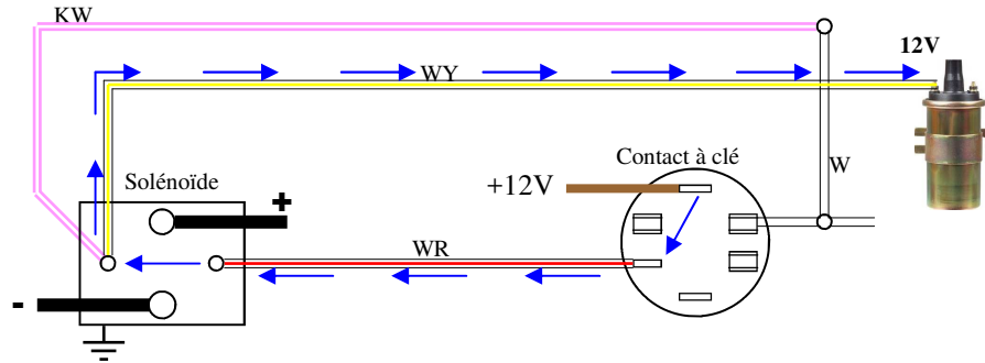
Schéma A position démarrage (Start)
