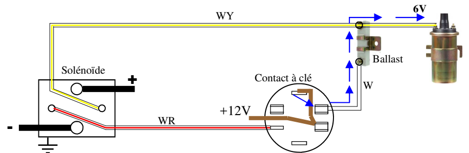
Schéma avec résistance ballast position marche (Ignition)
