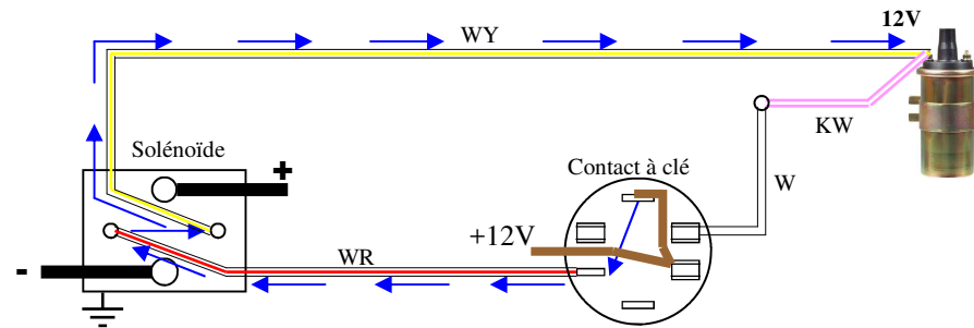
Schéma B position démarrage (Start)
