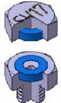
DIN 892 Magnet – Schraubenkopf Zum schnellen Vortäuschen einer Verschraubung auch von hinten idem des 2 cotés
