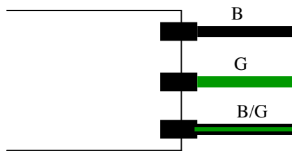
Moteur d'essuie-glace
